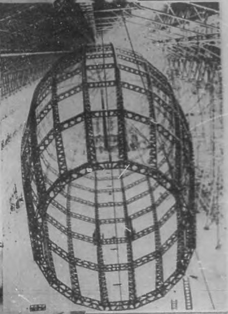
Armasón de acero del gigantesco Scythian que la Gran Bretaña está construyendo en Howden. Se llamará el K-100 y tendrá 700 pies de longitud, con un diámetro máximo de 130 pies. Su desplazamiento será de 150 toneladas y podrá alcanzar una velocidad de 32 millas por hora.
